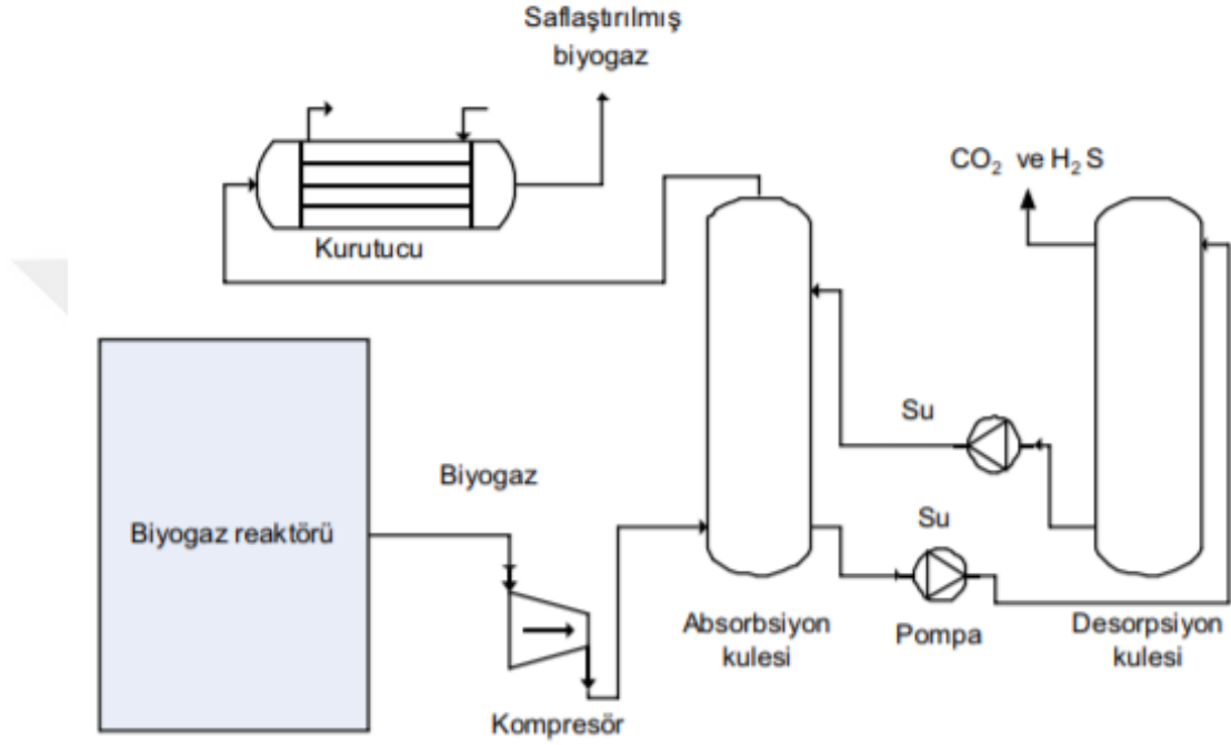
Şekil 3.1 : Su ile yıkama ünitesi
