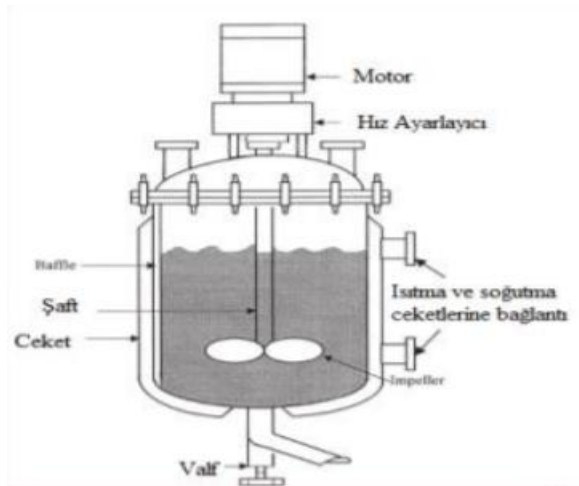
Şekil 2.3 : Kesik beslemeli tip reaktör
