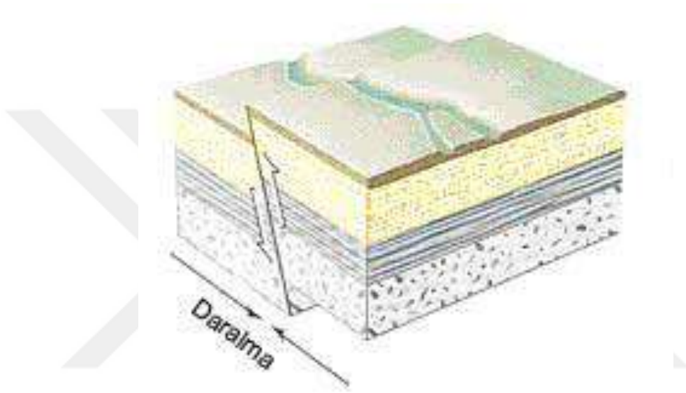
Şekil 1.11: Ters Atımlı Fay
