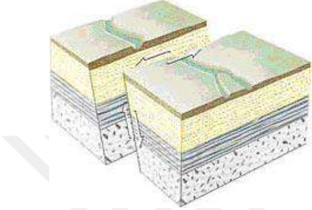
Şekil 1.12: Oblik Fay Türü
