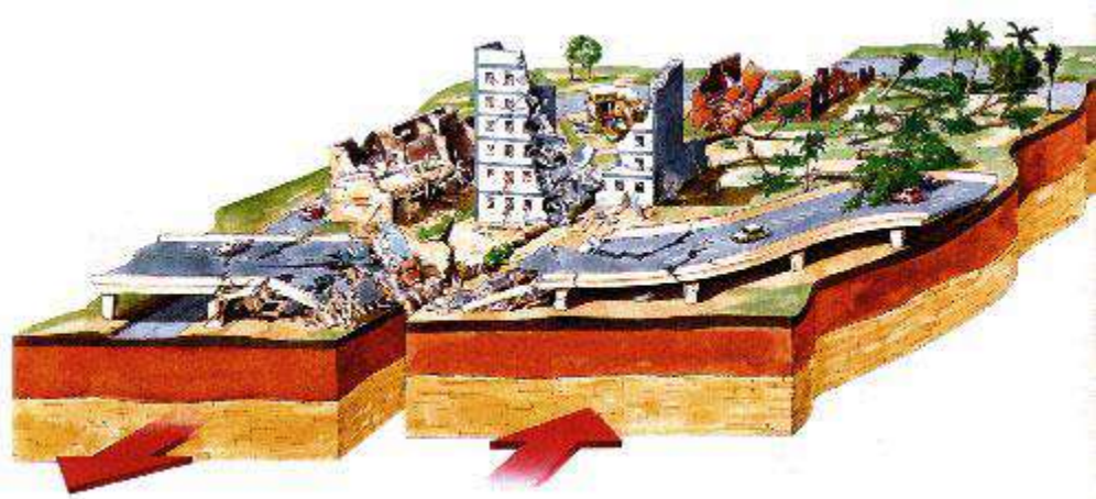
Şekil 1.3: Tektonik Deprem Oluşumu
