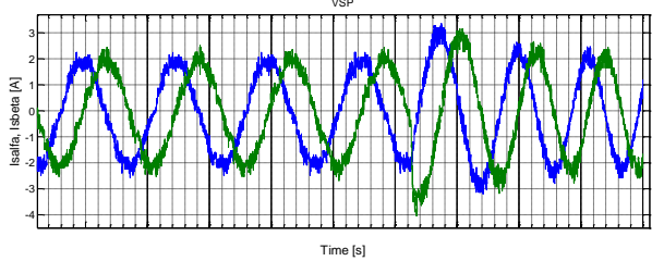
Şekil 14. T_L=0\text{Nm} iken ve \omega = 2000\text{dev/dk} 'dan 2800\text{dev/dk} hızına değiştirildiğinde a) I_{s_{abc}} , b) I_{s\alpha}, I_{s\beta}
