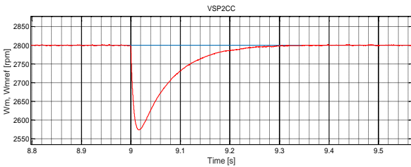
Şekil 7. \omega=2800\text{dev/dk} hızda, T_L=0\text{Nm} 'den 8\text{Nm} 'ye yük momentini ve hız değişikimi
