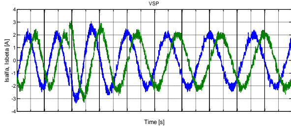
Şekil 12. T_L=0\text{Nm} iken ve \omega=2800\text{dev/dk} 'dan 2000\text{dev/dk} hızına değiştirildiğinde a) I_{s_{abc}} b) I_{s\alpha}, I_{s\beta}
