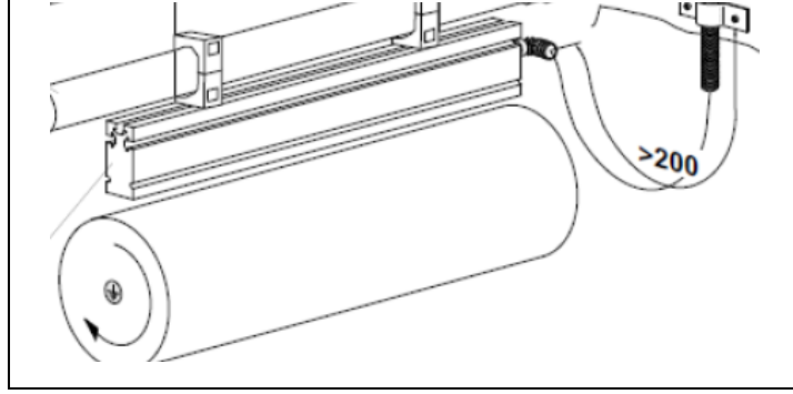
Şekil 5.10: Baskı Kauçuğu ve ESA Elektrot [15]
