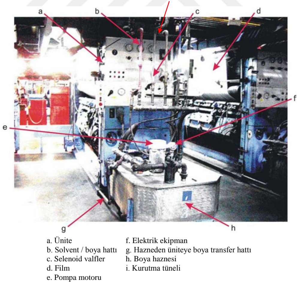
Şekil 5.1 : Baskı Ünitesi [4]
