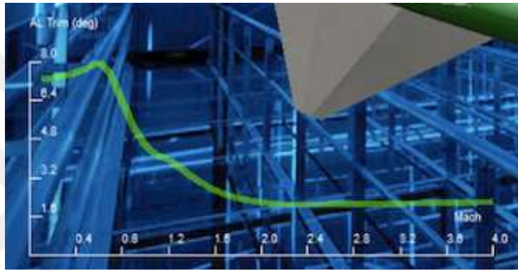
Şekil 4.12: Atgm_1 Füzesinin Hücum Açısı Katsayısı
