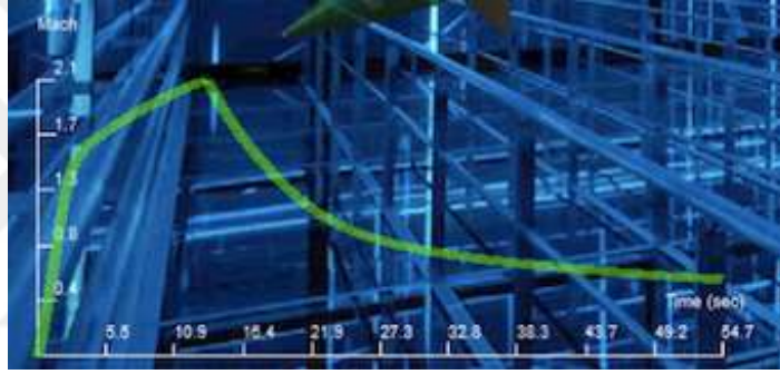
Şekil 4.57: Low Drag_8 Füzusunin Statik Test Mach Sayısı
